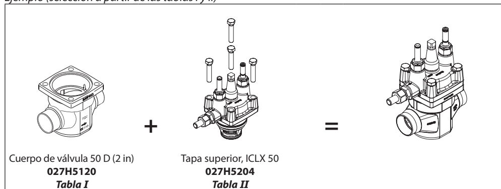
Cuerpo de válvula ICV 50 con distintos tipos de conexiones
